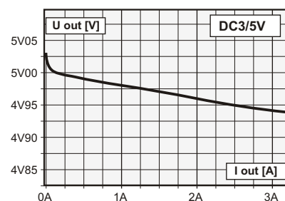
Typowy przebieg napięcia wyjściowego w funkcji prądu obciążenia Uwe = +15V, Uwy = +5V
