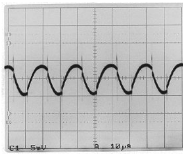
Typowy oscylogram napięcia na wyjściu przetwornicy DC3 dla: Uwe = +15V, Uwy = +5V, Iwy= 3.0A
